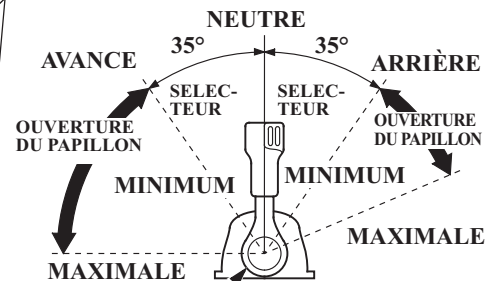
Levier de télécommande
