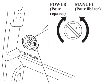
Soupape de décharge manuelle
