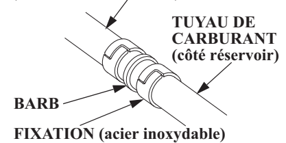
ASSEMBLAGE DU TUYAU DE CARBURANT (modèle équipé (côté moteur hors-bord))
