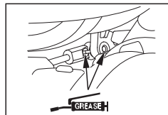
TIGE DU PAPILLON DES GAZ/ LIEN
