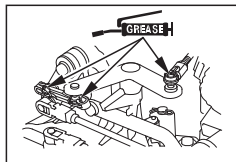
LEVIER D'ACCÉLÉRATEUR/ LIEN/PIVOT/PLAQUE
