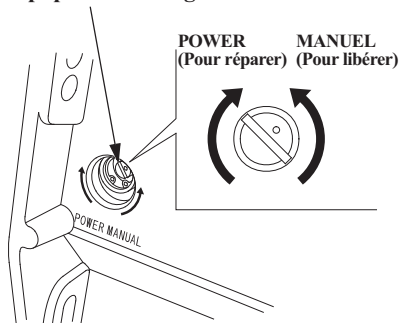
Soupape de décharge manuelle
