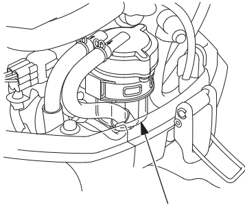
SEPARATEUR D'EAU
