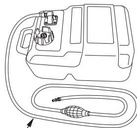
CONDUITE D'ESSENCE
